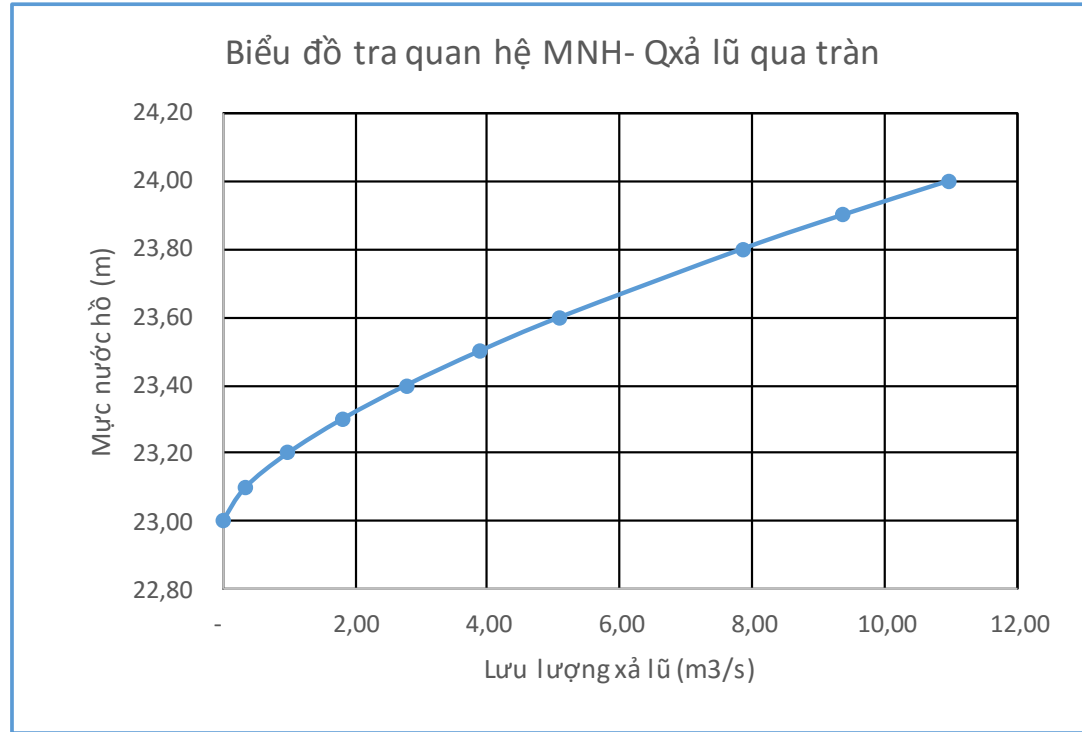
Bảng PL 3.4: Bảng tra quan hệ mực nước hồ ~ Q xả tràn tự do
